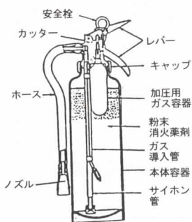
(加圧容器内蔵)
