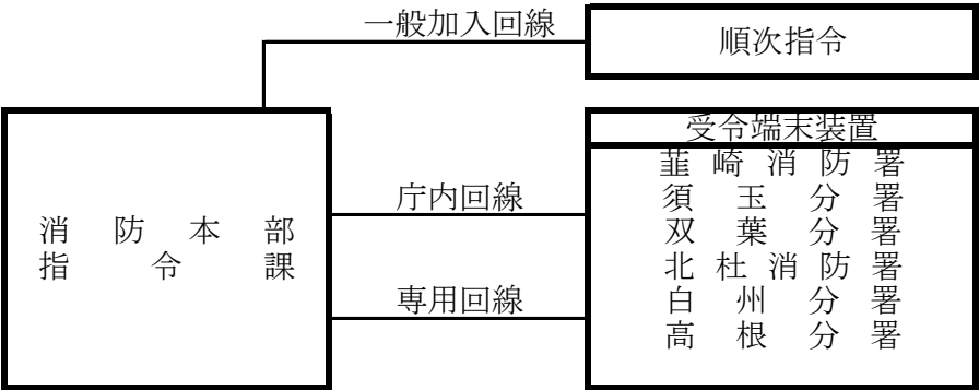
指令回線系統図
